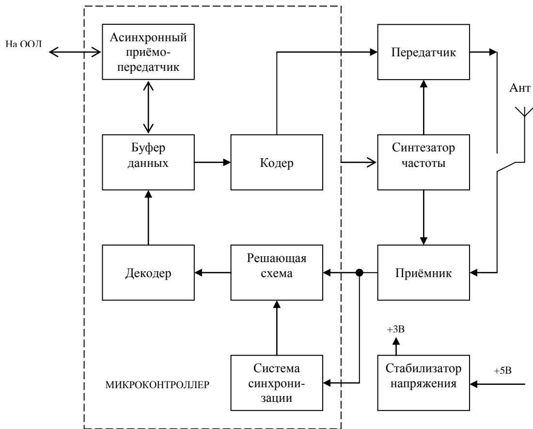
Рис. 2. Функциональная схема радиомодема
