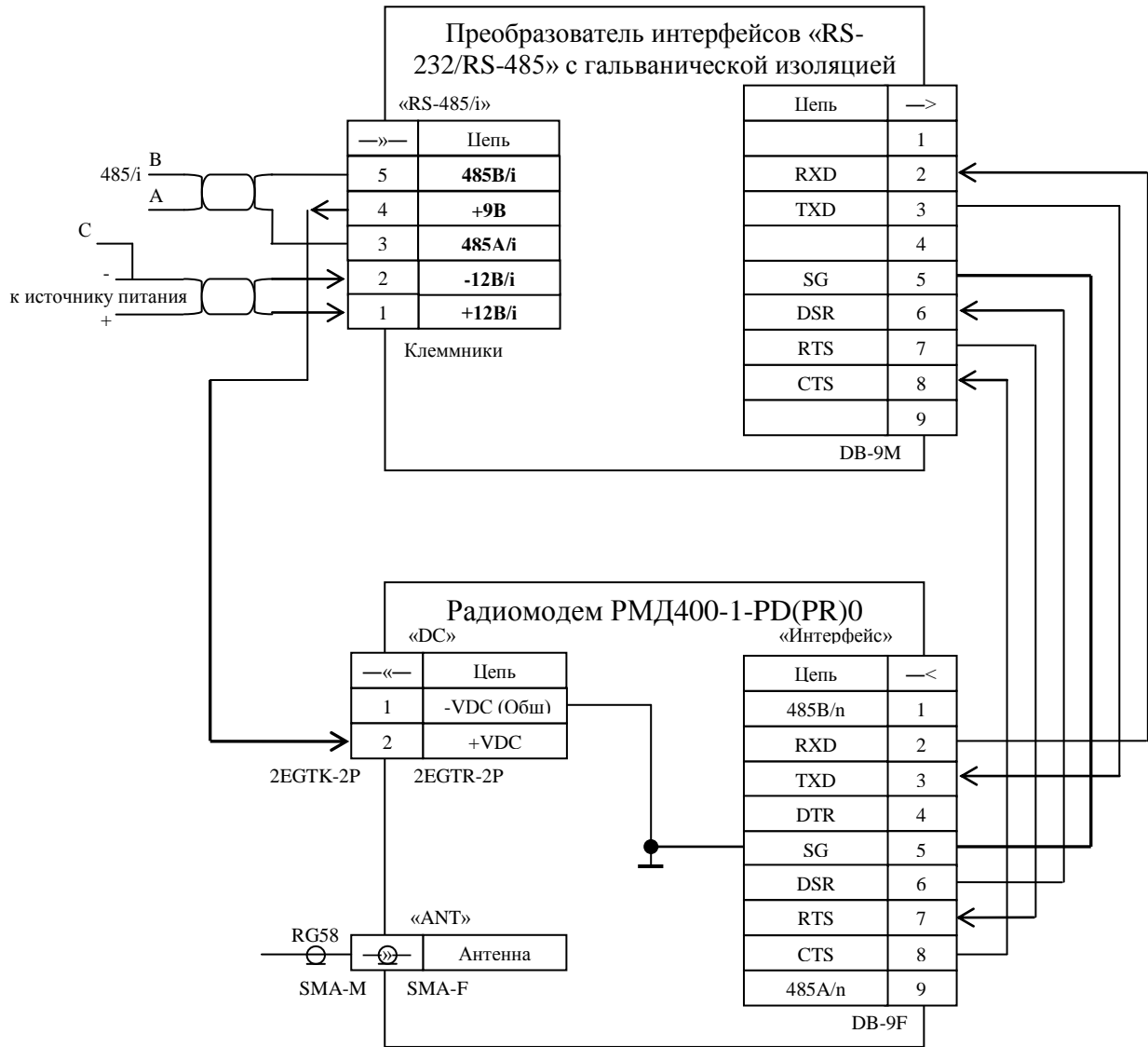
Рис.16 Схема соединения и внешнего подключения вариантов радиомодема РМД400-1-PD(PR)5 в режиме связи через интерфейс RS-485/i (с гальванической изоляцией)
