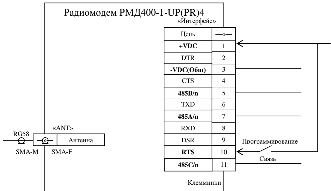
Рис.10 Схема подключения вариантов радиомодема РМД400-1-UP(PR)4 в режимах связи и программирования через гальванически неизолированный интерфейс RS-485
