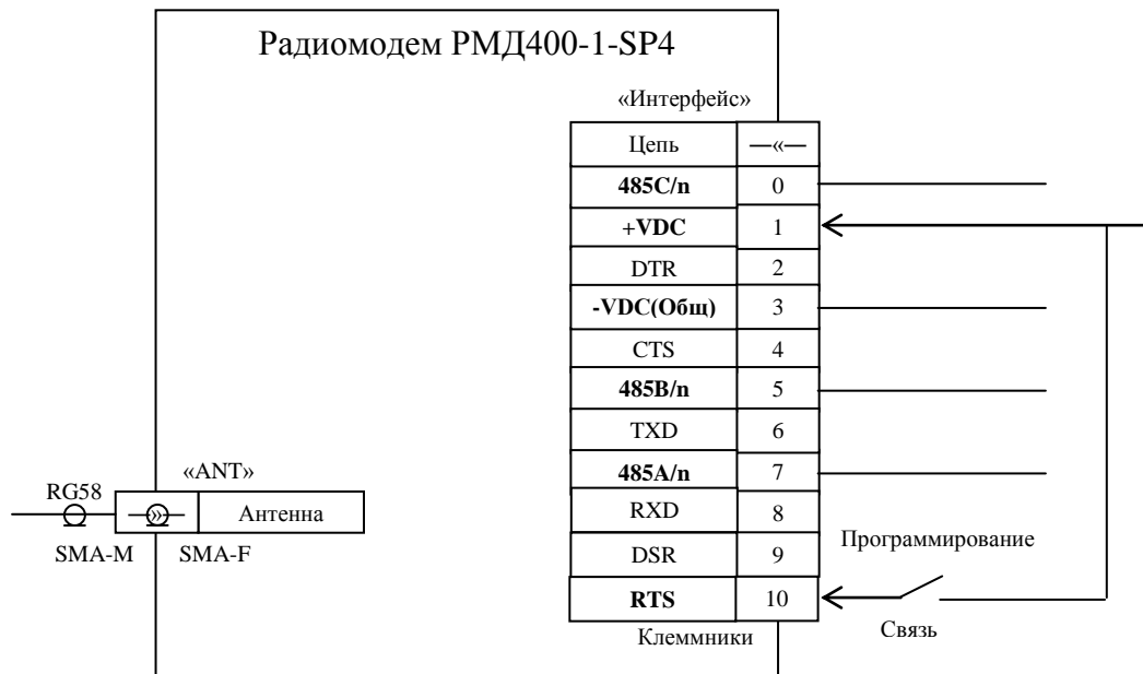
Рис.12 Схема подключения радиомодема РМД400-1-SP4 в режимах связи и программирования через гальванически неизолированный интерфейс RS-485
