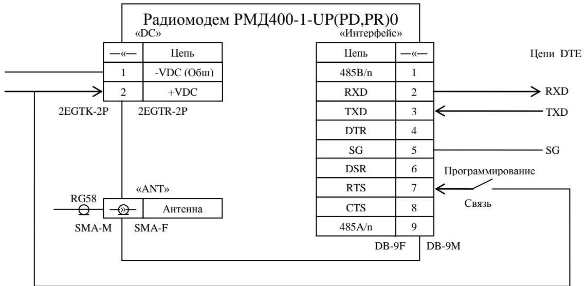
Рис.8 Схема подключения вариантов радиомодема РМД400-1-UP(PD,PR)0 с разъёмом DB-9F в режимах связи и программирования через интерфейс RS-232
