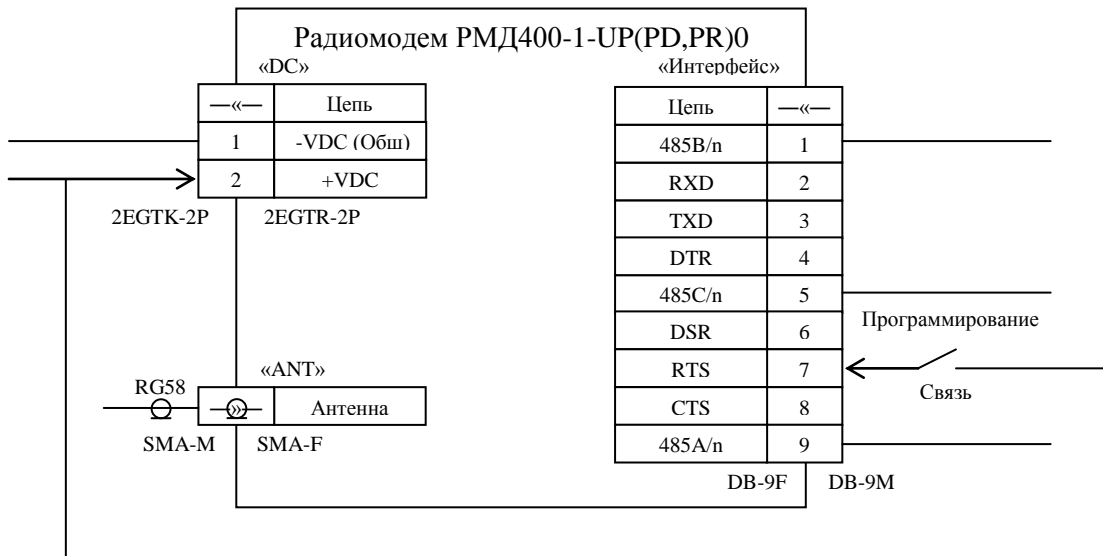
Рис.9 Схема подключения вариантов радиомодема РМД400-1-UP(PD,PR)0 с разъёмом DB-9F в режимах связи и программирования через интерфейс RS-485
