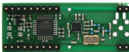
Рис.1 Внешний вид радиомодема РМД400-1-ОЕМ
