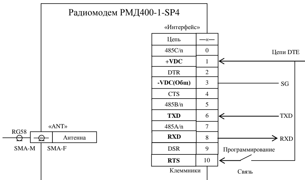
Рис.13 Схема подключения радиомодема РМД400-1-SP4 в режимах связи и программирования через интерфейс RS-232
