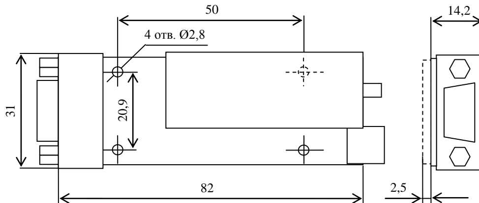
Рис.21 Габаритный чертёж бескорпусного варианта радиомодема РМД400-1-UP0
