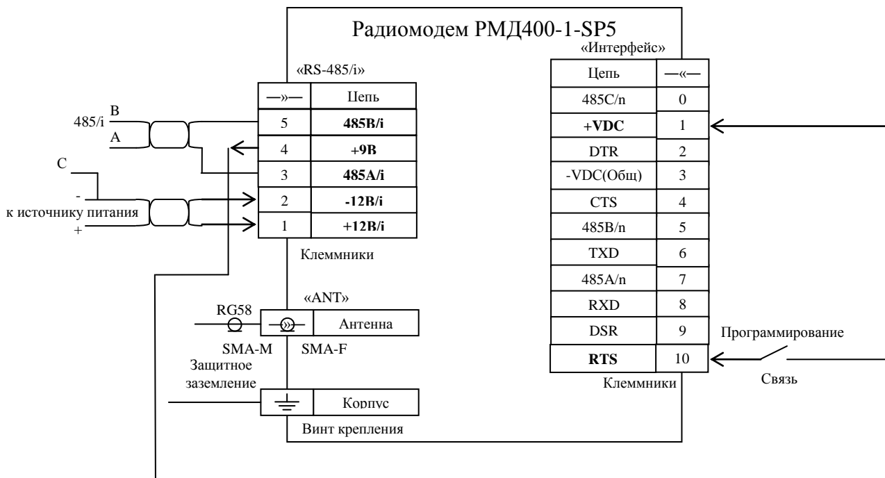
Рис. 14 Схема подключения радиомодема РМД400-1-SP5 в режимах связи и программирования через гальванически изолированный интерфейс RS-485
