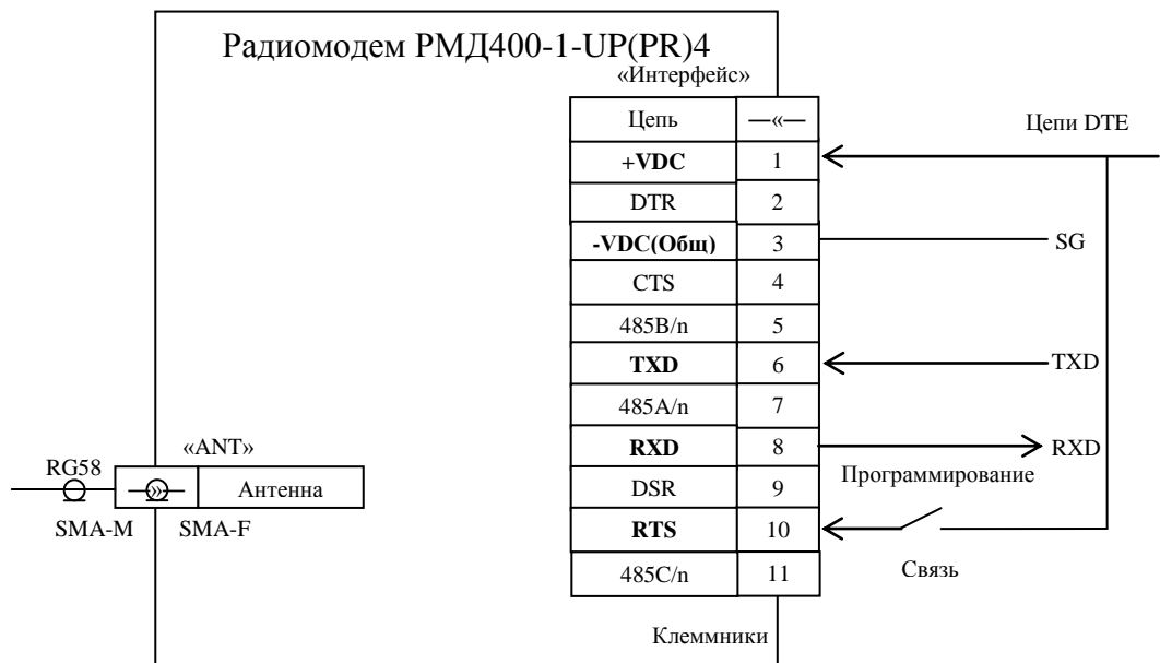
Рис.11 Схема подключения вариантов радиомодема РМД400-1-UP(PR)4 в режимах связи и программирования через интерфейс RS-232
