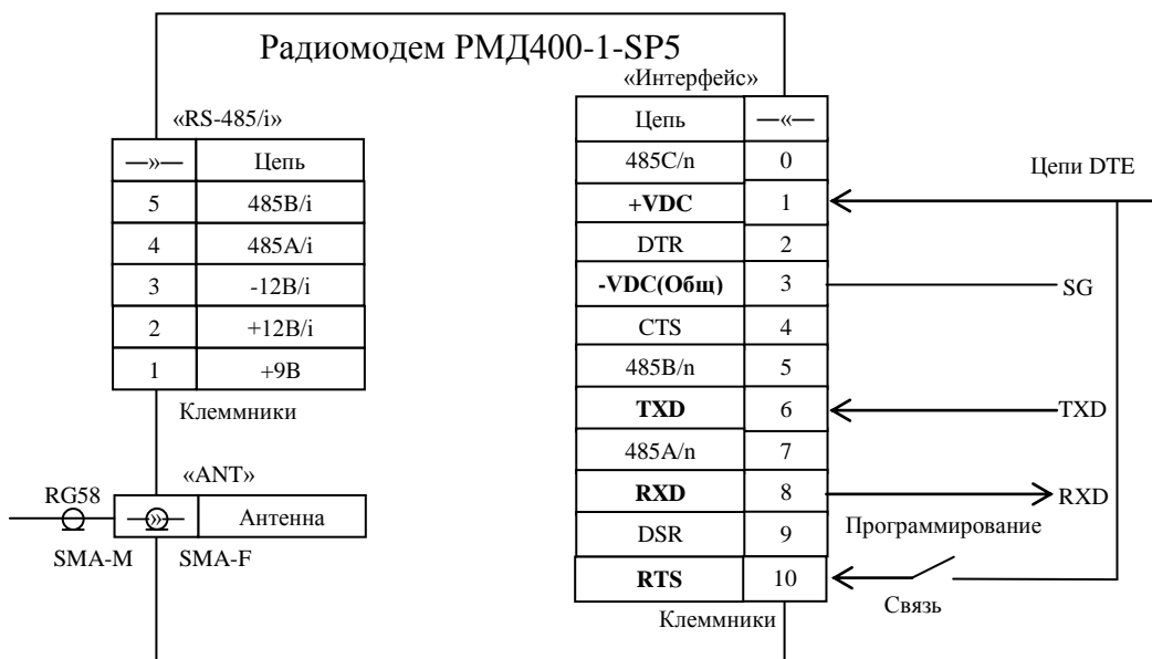
Рис. 15 Схема подключения радиомодема РМД400-1-SP5 в режимах связи и программирования через интерфейс RS-232
