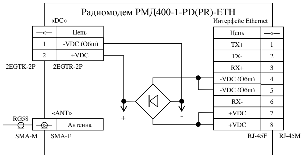
Рис.17 Схема подключения вариантов радиомодема РМД400-1-PD(PR)-ETH
