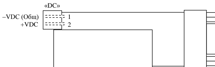
Рис.18 Схема расположения разъёма питания «DC» и его контактов (цепей) на плате адаптера интерфейсов
